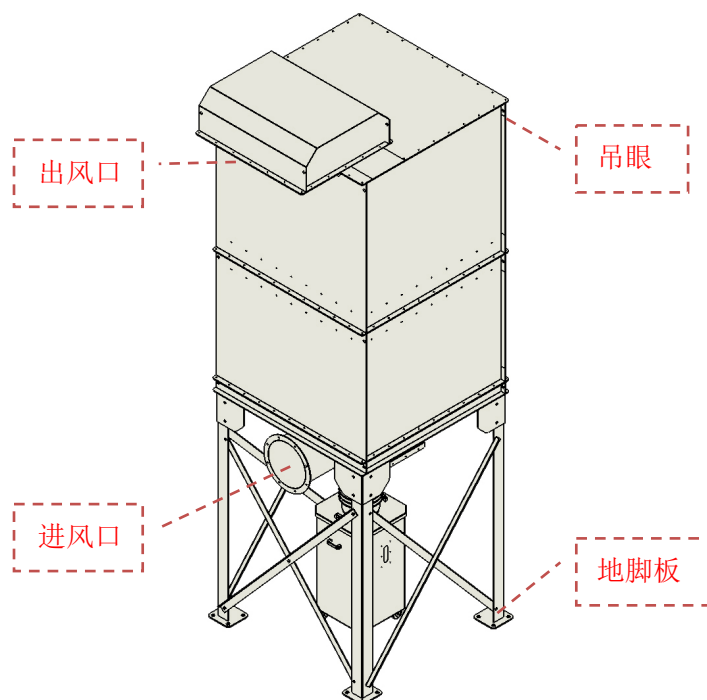
后视图
