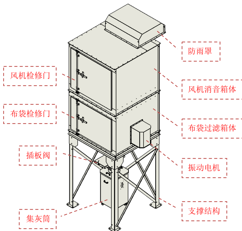
前视图
